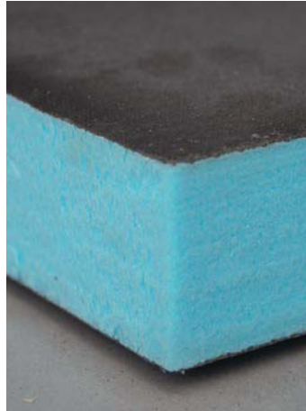
Die beidseitige Spezialbeschichtung des Duschboards erlaubt ein direktes Einkleben, Rundumabdichten und Befliesen des Boards.
